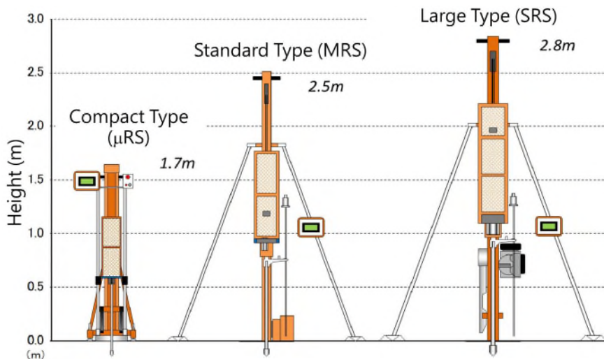
図：PDC調査で使用する3種類の動的貫入試験装置
